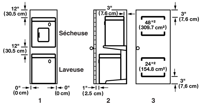
1. Encastrement 2. Vue latérale - placard ou endroit exigü 3. Porte de placard avec ouvertures d'entrée d'air
